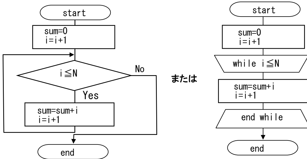
図 1-4 while 文による整数の和
